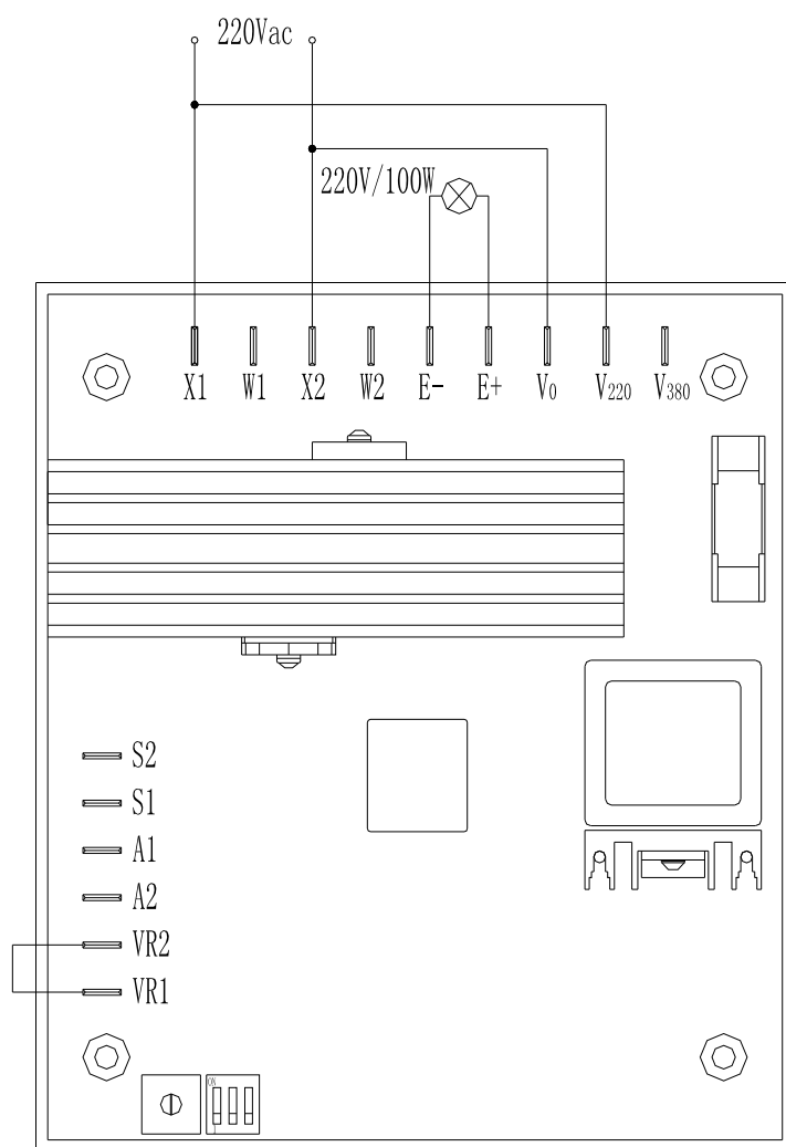
图 3 性能检测接线图
